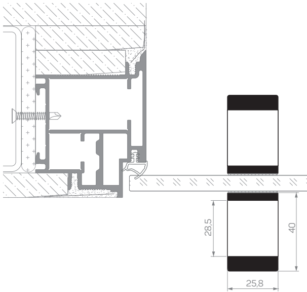
Rys. tech.: Zwymiarowany pochwyt
